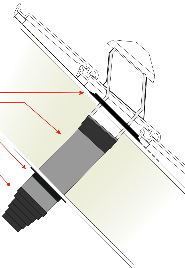
universele inbouwmanchet Ø 340 mm
